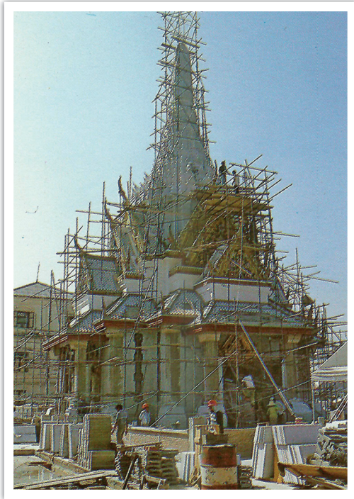
(ภาพเหตุการณ์) อาคารศาลหลักเมือง ขณะดำเนินการก่อสร้าง
