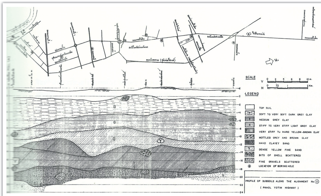
แผนผังจากวิศวกรรมสถานแห่งประเทศไทย ในพระบรมราชูปถัมภ์ : ข้อมูลสภาพดินบริเวณ ลุ่มแม่น้ำเจ้าพระยาตอนล่าง
