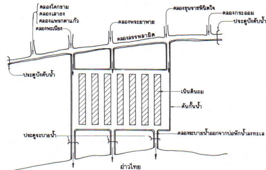
แผนผังแสดงระบบระบายน้ำ
