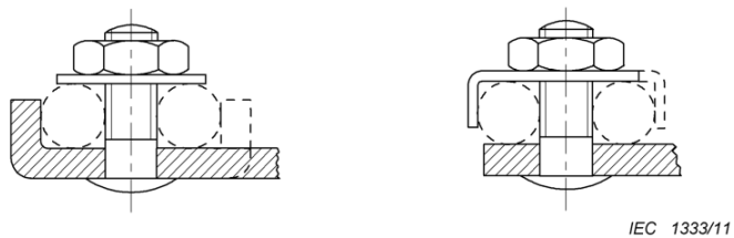
c) Stud terminals
