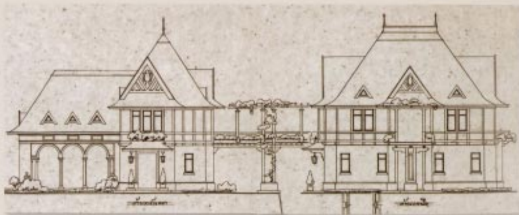
แบบแปลนพระตำหนักมารีราชรัตบัลลังก์ ม.จ.อิทธิเทพสรรค์ กฤดากร ผู้เขียนแบบ พ.ศ. ๒๔๕๗
