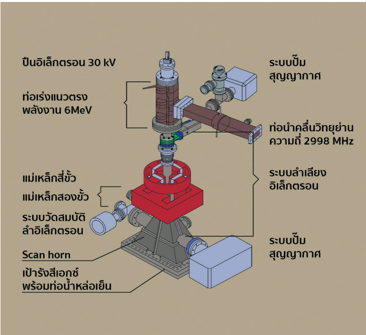
เครื่องเร่งอนุภาคเพื่อการเกษตร (ภาพซ้าย) เจ้าหน้าที่เทคนิคของสถาบันวิจัยแสงซินโครตรอน (องค์การมหาชน) กำลังติดตั้งระบบเครื่องเร่งอนุภาคแนวตรงเพื่อการอาบผลไม้ให้ปลอดเชื้อ (ภาพขวา) ไดอะแกรมของระบบเครื่องเร่งแนวตรงดังกล่าว (ภาพเมื่อ มกราคม ค.ศ. 2020)
