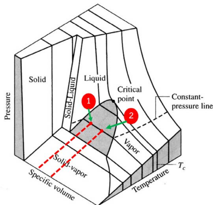
รูปที่ 4-3 พื้นผิว P-v-T
