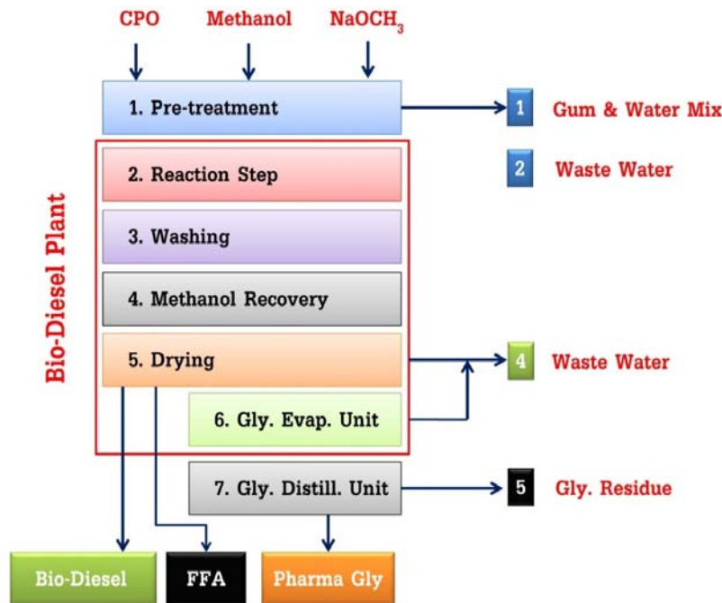
รูปที่ 15-12 แสดงกระบวนการผลิตไบโอดีเซล ด้วยปฏิกิริยาทรานเอสเทอร์ริฟิเคชัน
