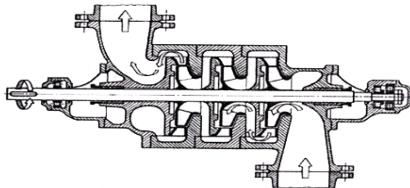
รูปที่ 11-17 ปั๊มน้ำแบบแรงเหวี่ยงประเภทความกดดันสูง หรือหลายสแตจ
