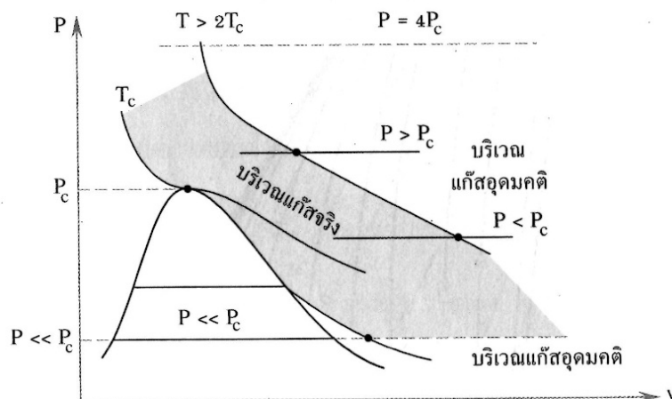
รูปที่ 4-7 สภาวะของแก๊สอุดมคติ (ที่มา: อุณหพลศาสตร์ 1 [รศ.มนตรี พิรุณเกษตร, 2550])
