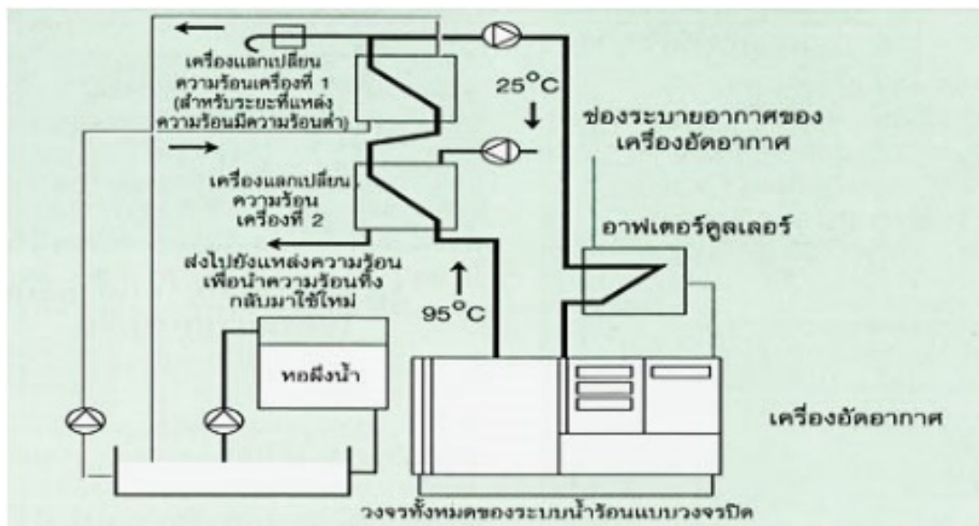
รูปที่ 1-7 รูปแสดงระบบการนำความร้อนทิ้งกลับมาใช้ใหม่
