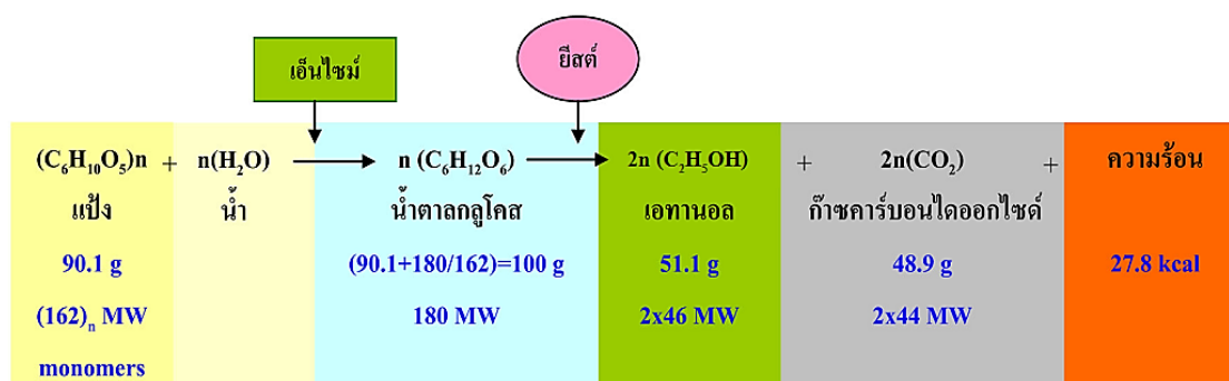
รูปที่ 15-8 แสดงสมการทางเคมีของการเปลี่ยนแป้งเป็นเอทานอล
