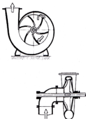
รูปที่ 11-11 ปั้มน้ำแบบแรงเหวี่ยงประเภทความกดดันต่ำ
