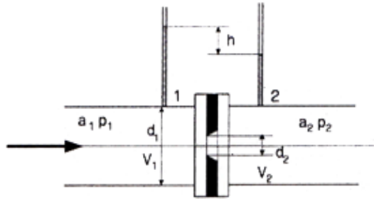
รูปที่ 11-8 อุปกรณ์การวัดแบบออร์ฟิซมิเตอร์
