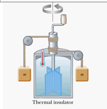
รูปที่ 4-9 กฎข้อที่หนึ่งของอุณหพลศาสตร์
