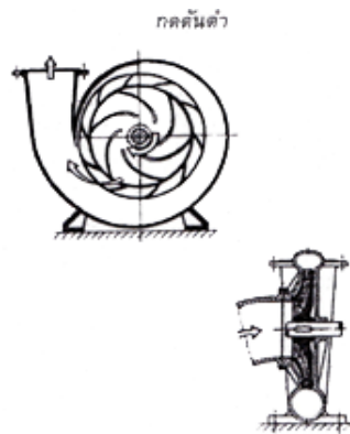
รูปที่ 11-16 ปั๊มแรงเหวี่ยงประเภทความกดดันปานกลาง
