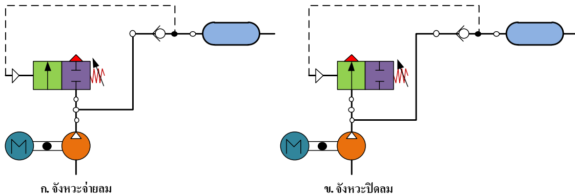
รูปที่ 1-13 การควบคุมแบบระบายลมอัด Exhaust Regulation
