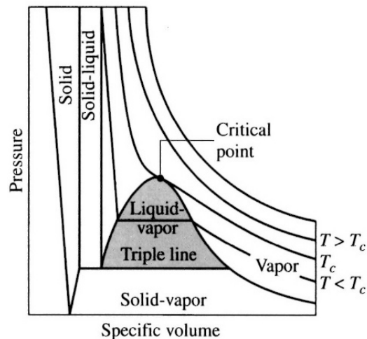
รูปที่ 4-5 พื้นผิว P-v-T ในแนวตั้งฉากกับระนาบ P-v
