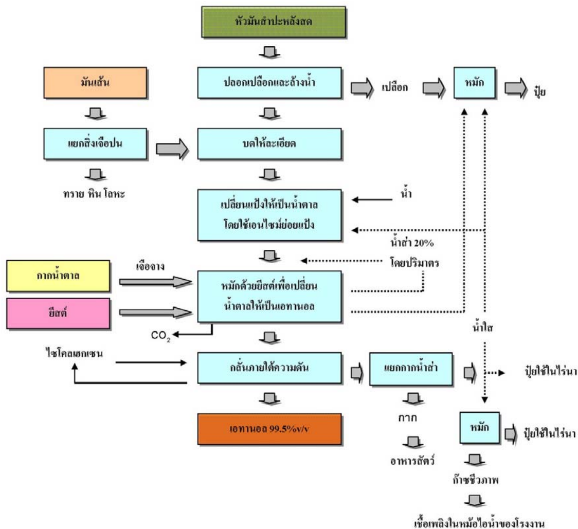
รูปที่ 15-7 แผนผังแสดงขั้นตอนการผลิตเอทานอลจากมันสำปะหลังและอ้อยในโรงงานต้นแบบของ วว.
