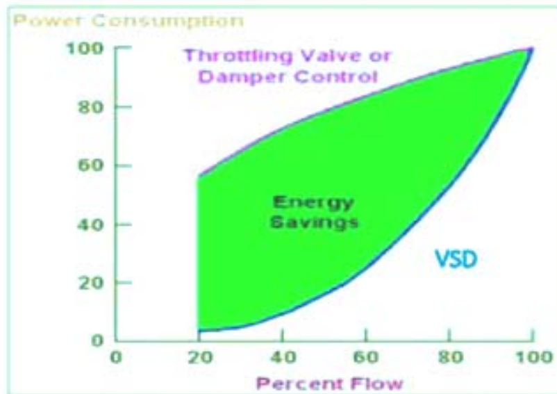
รูปที่ 11-23 แสดงเปรียบเทียบการใช้พลังงานระหว่างการใช้อวาล์วควบคุมการไหล และการใช้อุปกรณ์ควบคุมความเร็วมอเตอร์
