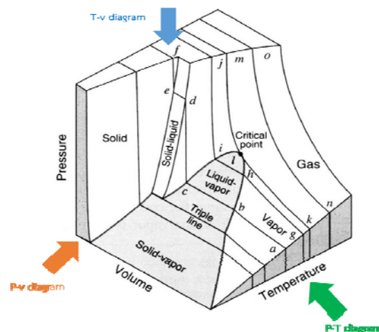
รูปที่ 4-2 สมบัติของสารบริสุทธิ์สามารถอธิบายด้วยกราฟ 3 มิติ
