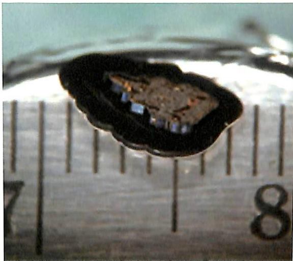
ภาพจากกล้องจุลทรรศน์แสดงคราสัญลักษณ์ บนแผ่นฐาน निकเกิลเทียบกับสเกลไม้บรรทัด (จีคละ 1 มิลลิเมตร)
