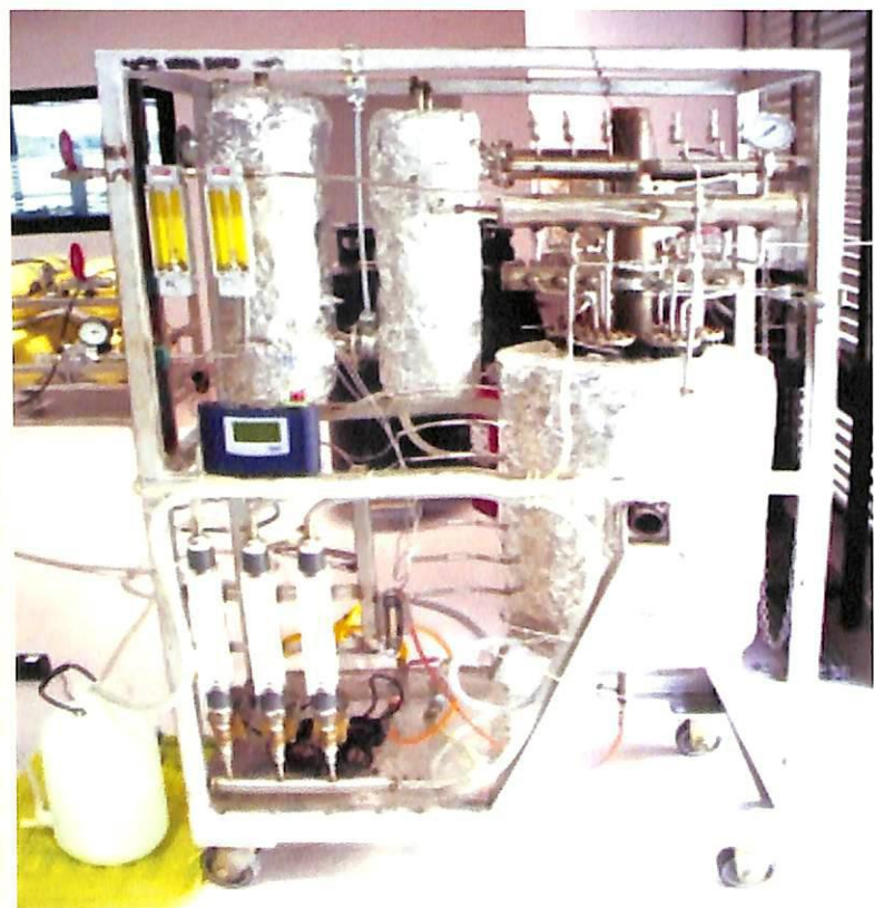
ชุดปฏิรูปก๊าซมีเทนจากก๊าซชีวภาพ เป็นก๊าซไฮโดรเจน
