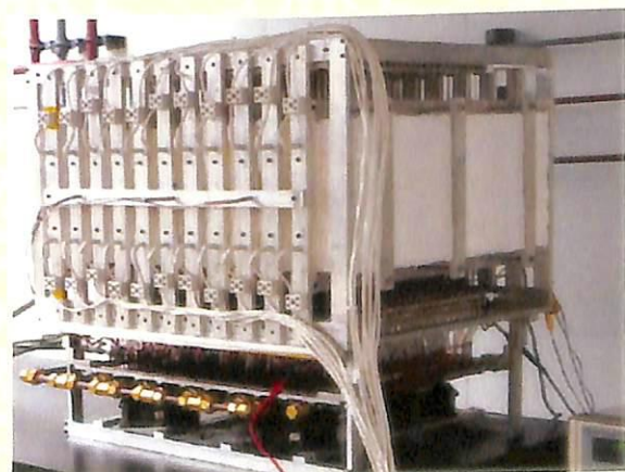
เซลล์เชื้อเพลิงแบบออกไซด์ของแข็ง
