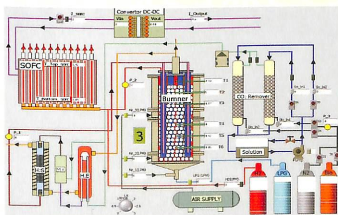
ส่วนประกอบต่างๆ สำหรับการผลิตไฟฟ้า จากเซลล์เชื้อเพลิงโดยใช้ก๊าซชีวภาพ
