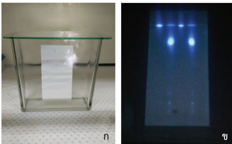
ภาพที่ 6.6 (ก) แผ่น TLC แขนในตัวทำละลาย (ข) การเรืองแสงฟลูออเรสเซนซ์ภายใต้แสง UV ที่แยกได้ด้วยวิธี TLC
