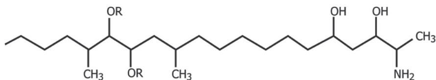
Fumonisin B 2
