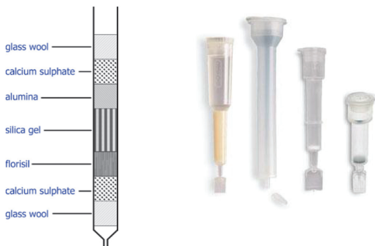
ภาพที่ 6.5 ส่วนประกอบและลักษณะของ minicolumn แบบต่าง ๆ
