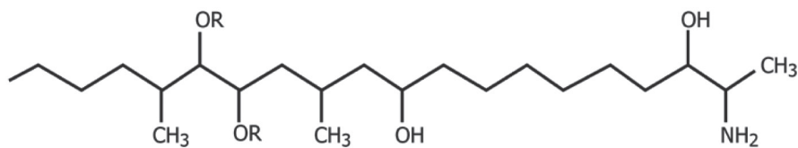
Fumonisin B 3
