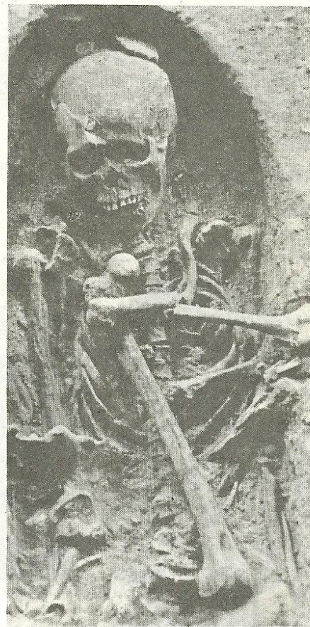
โครงกระดูกของมนุษย์ สมัยก่อนประวัติศาสตร์ที่โคกพลับ ต.โพหัก อ.บางแพะ ราชบุรี
