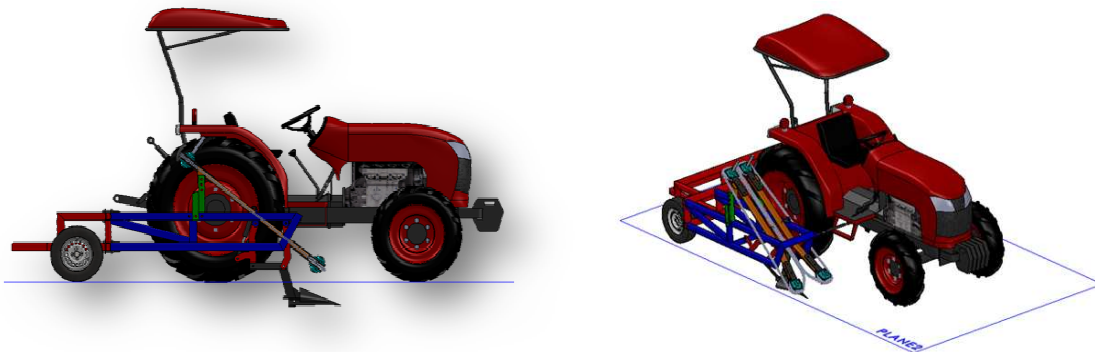
รูปแบบของเครื่องเก็บเกี่ยวมันสำปะหลังสำหรับรถแทรกเตอร์ขนาดเล็ก
