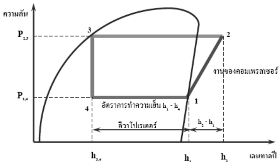
รูปที่ 3-10 แผนภาพความดัน-เอนทัลปีของวัฏจักรการทำความเย็นแบบอัดไอ
