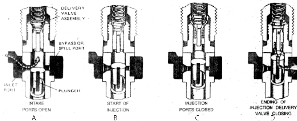
รูปที่ 2-26 แสดงลำดับขั้นตอนการทำงานของปั๊มฉีดน้ำมันเชื้อเพลิง
