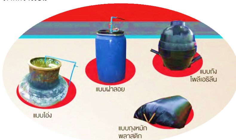
รูปที่ 14-6 การผลิตก๊าซชีวภาพภาคครัวเรือน
