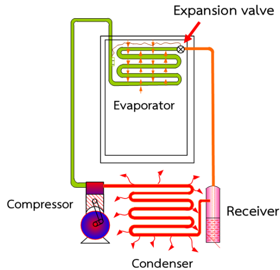
รูปที่ 3-5 อุปกรณ์หลักของระบบการทำความเย็นแบบอัดไอ
