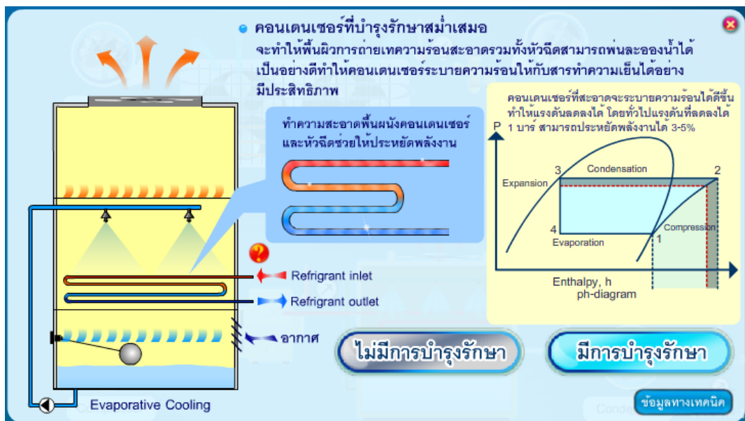
รูปที่ 3-25 การบำรุงรักษาอุปกรณ์คอนเดนเซอร์
