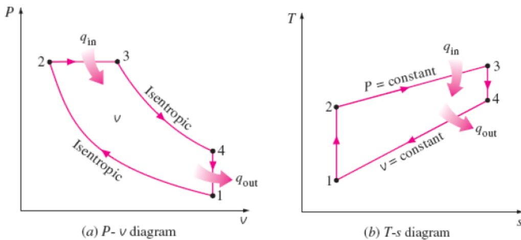
รูปที่ 2-5 วัฏจักรดีเซลตามทฤษฎี
