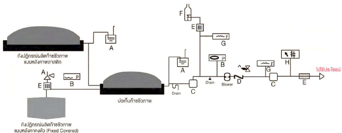
รูปที่ 14-18 อุปกรณ์เพื่อความปลอดภัยและแผนผังการติดตั้งอุปกรณ์ในระบบผลิตก๊าซชีวภาพ
