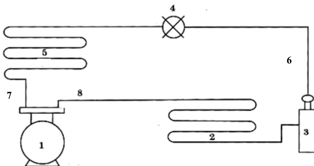
รูปที่ 3-2 แสดงวงจรทางกลระบบการทำความเย็นแบบอัดไอ
