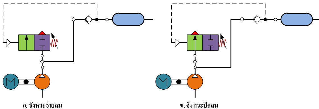
รูปที่ 2-9 การควบคุมแบบระบายลมอัด Exhaust Regulation
