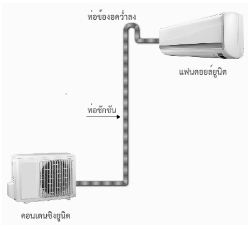
รูปที่ 3-18 การวางท่อทางเดินสารทำความเย็น กรณีที่ คอยล์เย็น สูงกว่า คอยล์ร้อน (ที่มา: วิศวกร วิศวกร และ สมชาย วิศวกร “เครื่องทำความเย็นและเครื่องปรับอากาศ”, พ.ศ. 2556)
