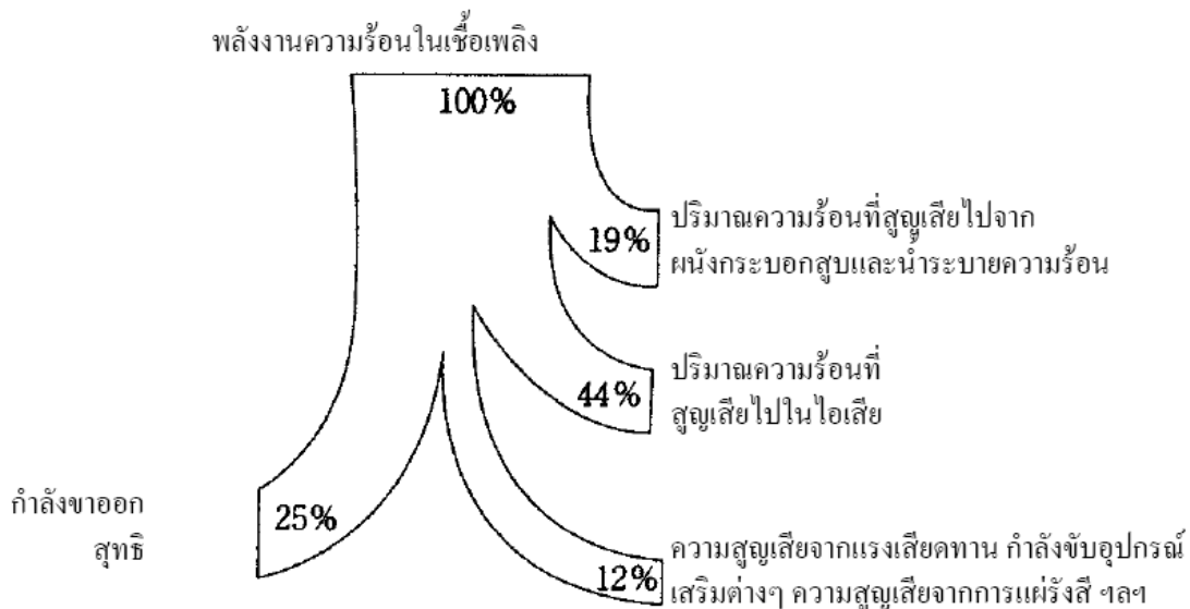
รูปที่ 2-27 ตัวอย่างสมดุลความร้อนของเครื่องยนต์ดีเซล
