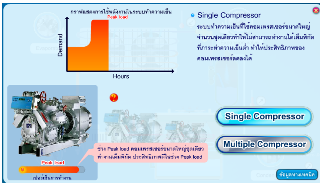
รูปที่ 3-22 แนวทางการประหยัดพลังงานในอุปกรณ์คอมเพรสเซอร์ แบบตัวเดียว
