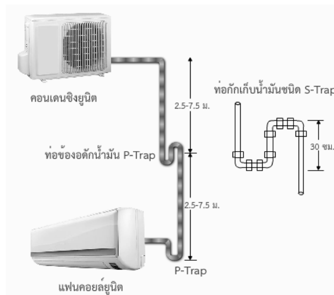
รูปที่ 3-17 การวางท่อทางเดินสารทำความเย็น กรณีที่ติดตั้ง คอยล์ร้อน สูงกว่า คอยล์เย็น (ที่มา: วิกิพีเดีย มโนน้อม และ สมชาย วนารักษ์ “เครื่องทำความเย็นและเครื่องปรับอากาศ”, พ.ศ. 2556)
