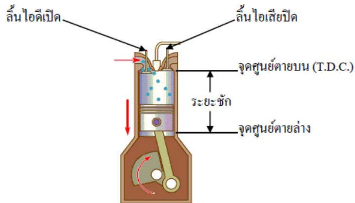
รูปที่ 2-11 จังหวะดูด
