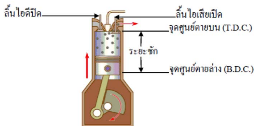
รูปที่ 2-14 จังหวะคาย
